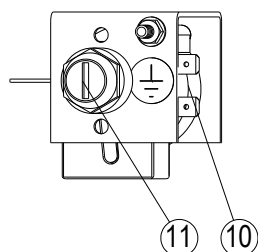
Ogranicznik temperatury poz. 10
