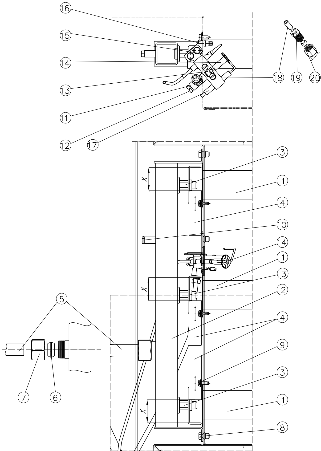
Rysunek 3 - Zespół palników i pilota
