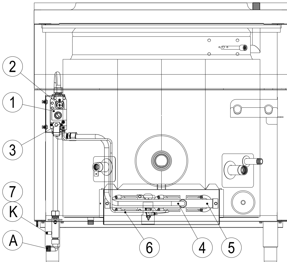
Rysunek 4a - Instalacja gazowa
